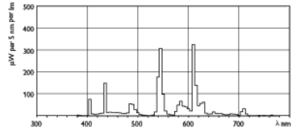
PL-L/835
