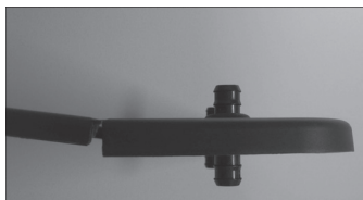
Installez les nouveaux connecteurs à accouplement droit dans les rondelles restantes
