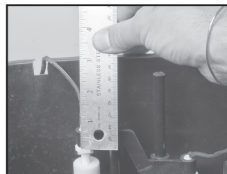
Interrupteur de flotteur supérieur 7,60 cm (3") sous la partie supérieure du récipient
