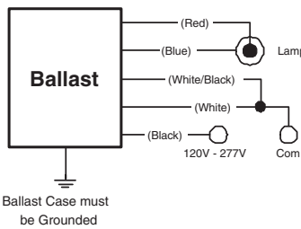
Wiring Diag. 2
