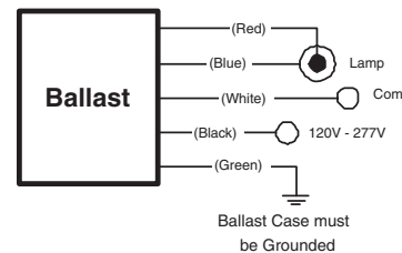
Wiring Diag. 3
