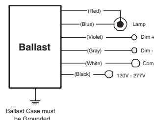
Wiring Diag. 6
