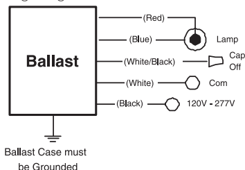
Wiring Diag. 1
