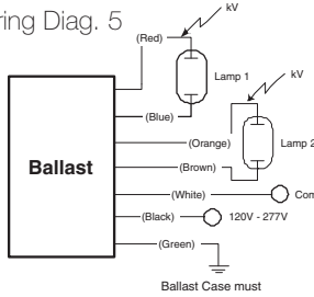
Wiring Diag. 5
