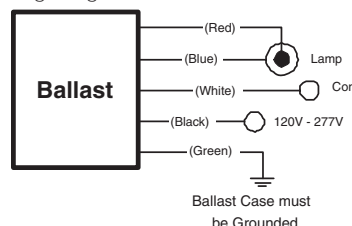
Wiring Diag. 3
