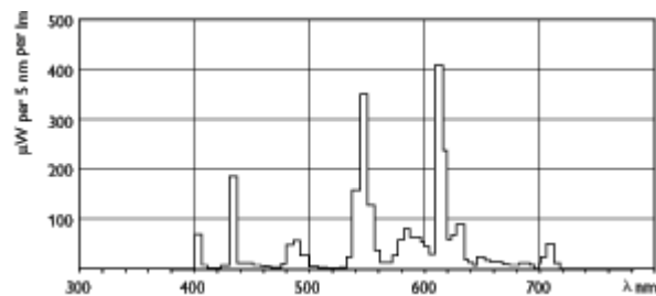
PL-L/830
